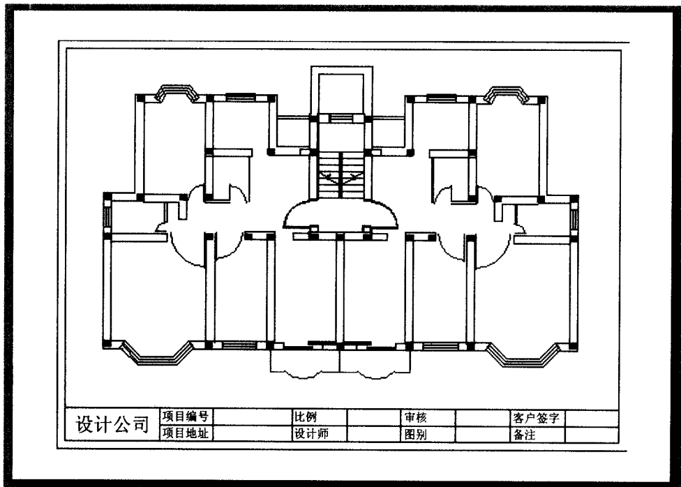
图 1-1-6 输出图形
