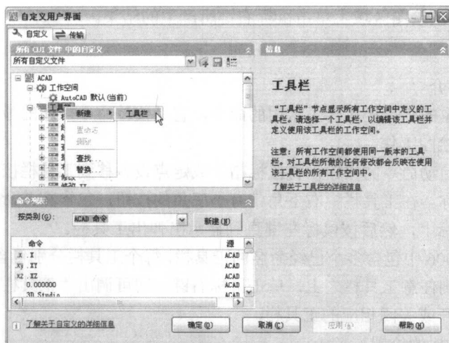
图 1-1-13 “自定义用户界面”（自定义）对话框
