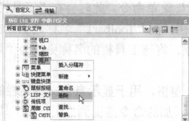
图 1-1-16 删除工具栏
