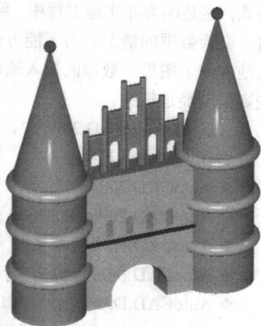
图 1-1-5 渲染图形
