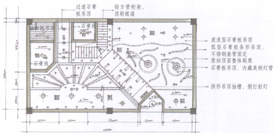
顶面布置图 1:50
