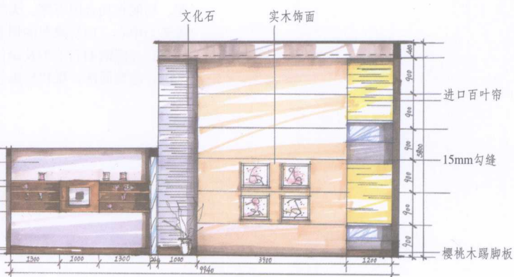
B向立面图 1:50
