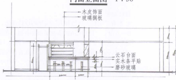
吧台立面图 1:50
