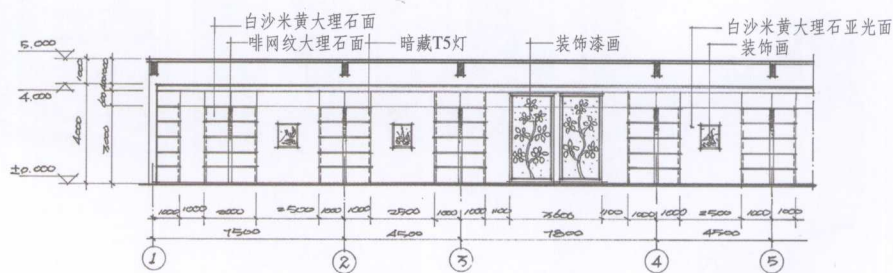
①~⑤轴立面 1:100
