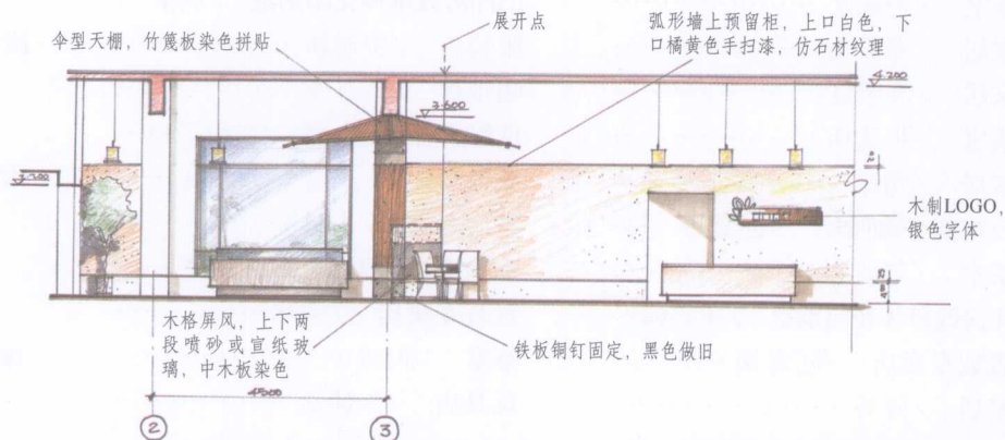
室内主立面图 1:50
