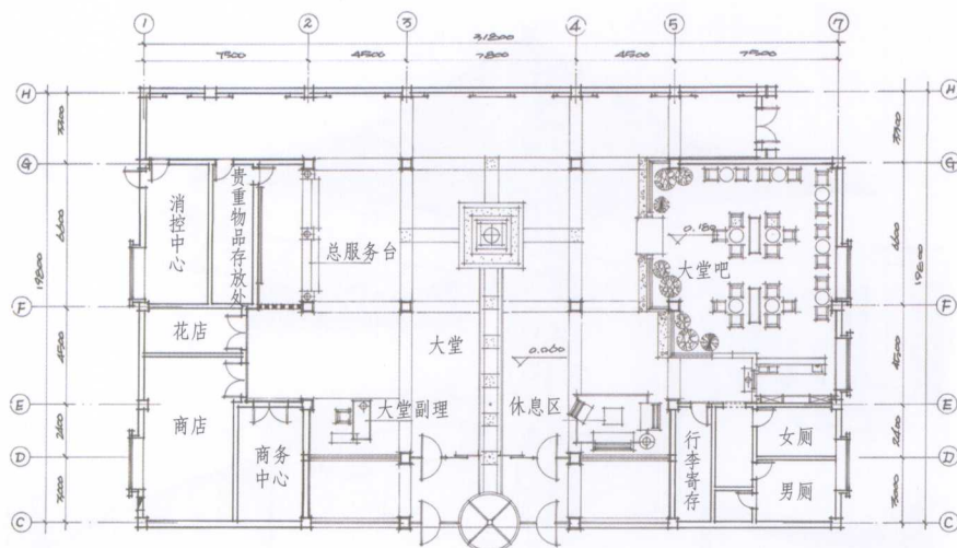
平面布置图 1:100
