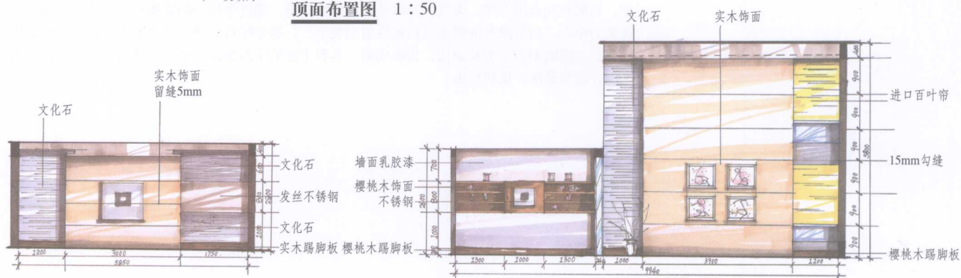
A向立面图 1:50
