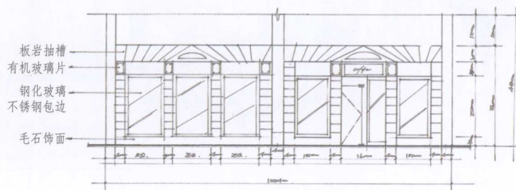
门面立面图 1:50
