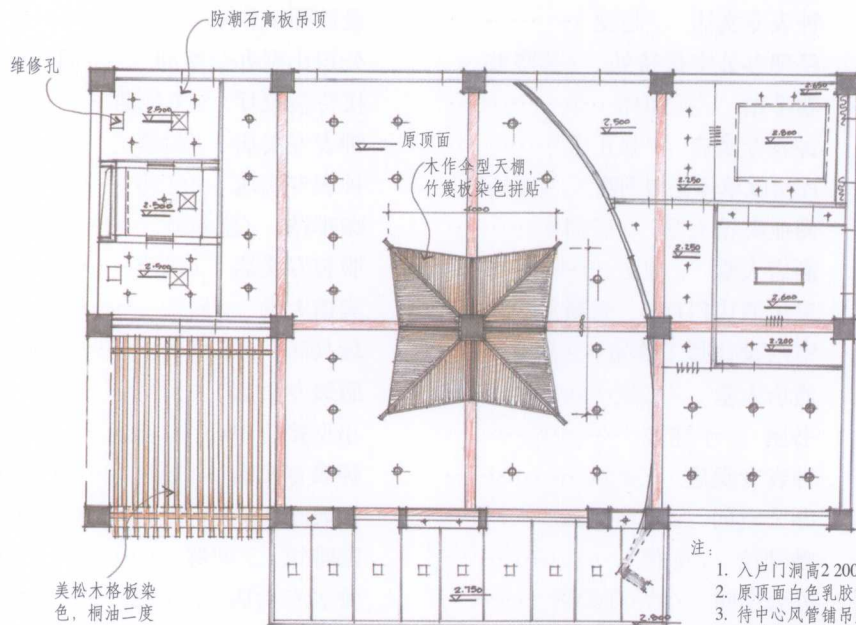
售楼处顶面图 1:50
