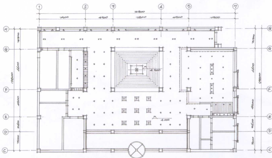
顶面布置图 1:100
