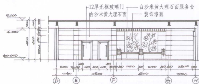
⑥~⑦轴立面图 1:100
