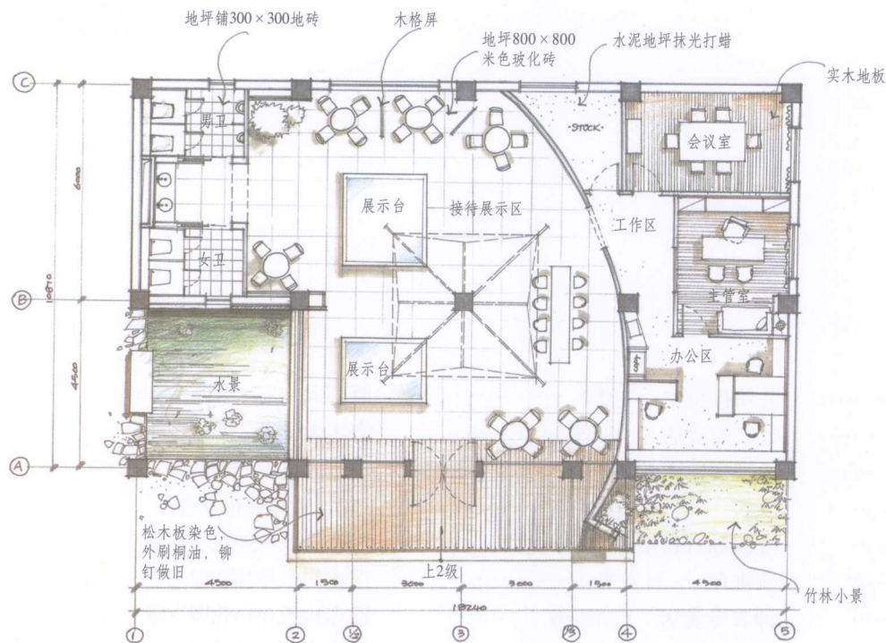
售楼处平面图 1:50
