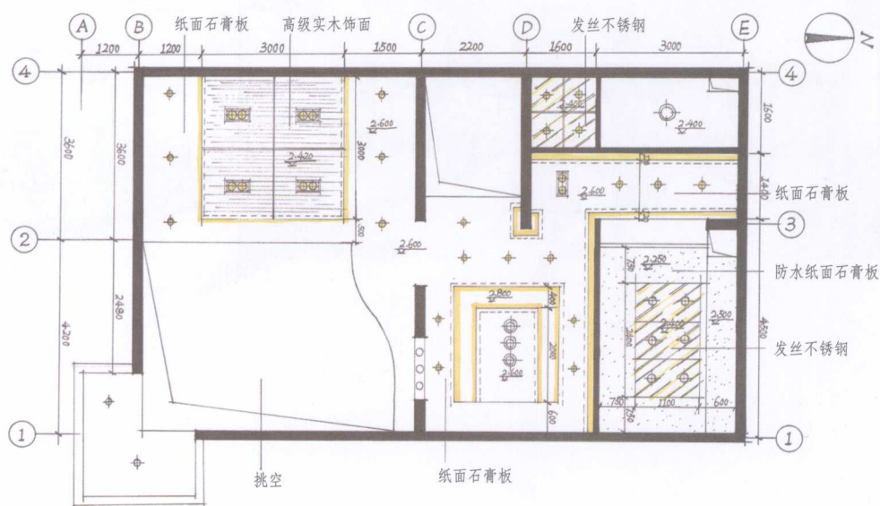
平面布置图 1:50
