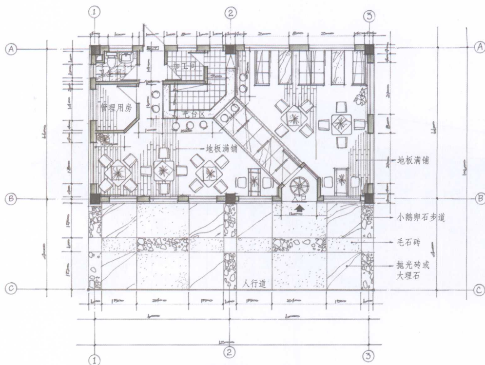
平面布置图 1:50
