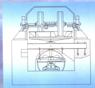
SH2750型湿碾机
