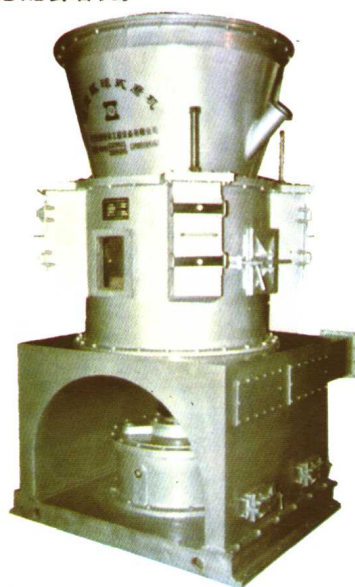
H63 型 H63A 型
