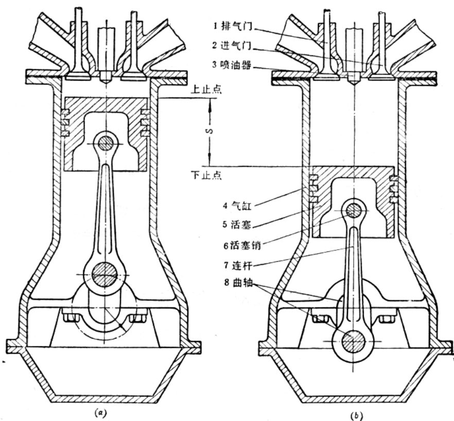
图1-1 单缸四行程柴油机简图
