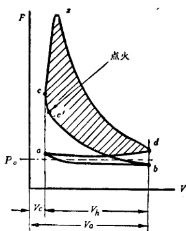
图1-5 四行程汽油机示功图
