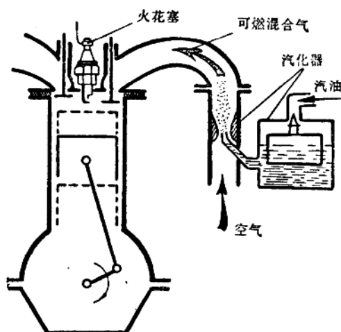
图1-4 单缸四行程汽油机简图
