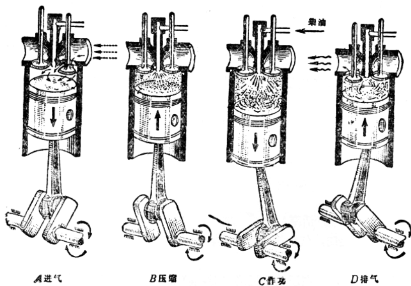
图1-2 单缸四行程柴油机的工作过程
