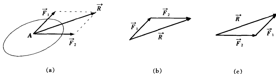
图 2-10 力的平行四边形法则
