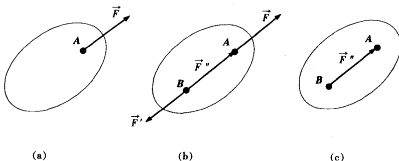
图 2-9 力的可传性
