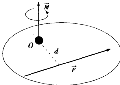
图 2-6 力对点的矩
