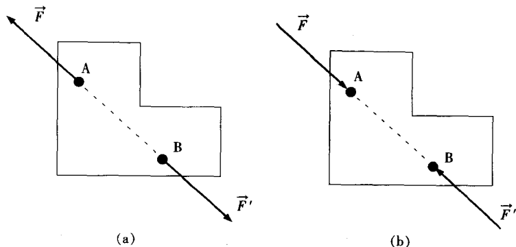
图 2-8 二力平衡
