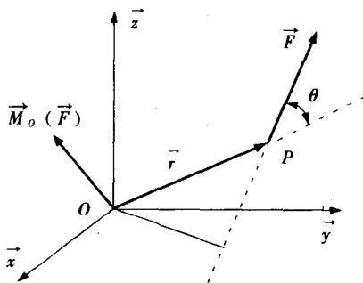
图 2-7 力对点的矩的叉积表示
