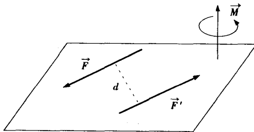
图 2-5 力 偶 矩
