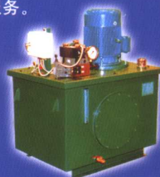
冶金环保设备用液压系统
