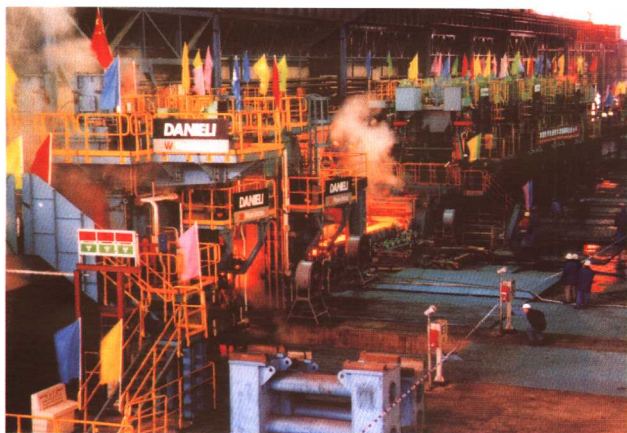
△ 一钢轧厂 1810mm 轧机生产线
