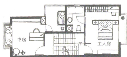
三楼平面图
