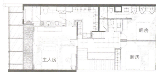
二楼平面图
