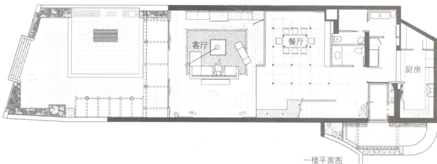
一楼平面图
