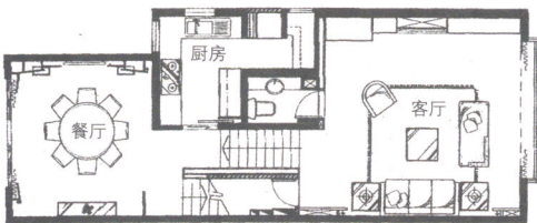
一楼平面图
