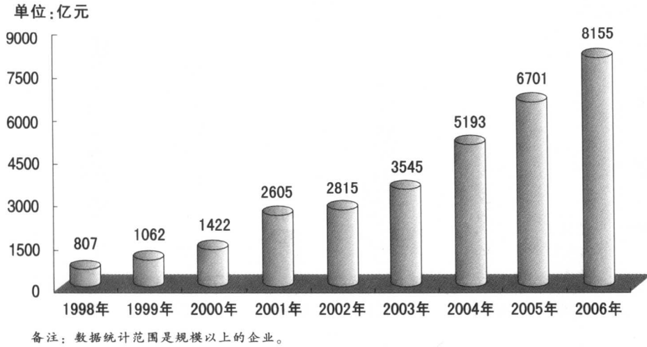
图 16 1998—2006 年电子信息产品制造业工业增加值完成情况
