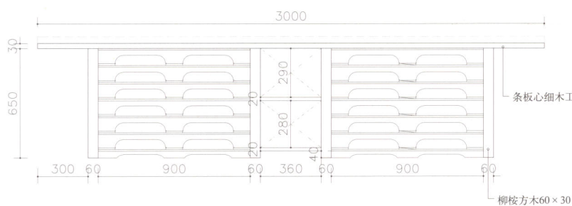
后视图
