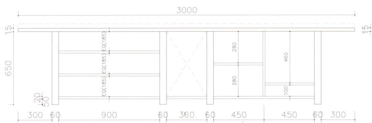
正视图
