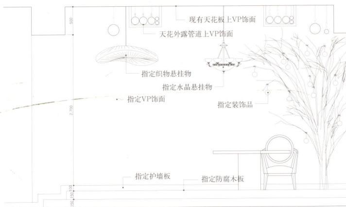
舞台细部图
