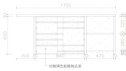
侧视图
