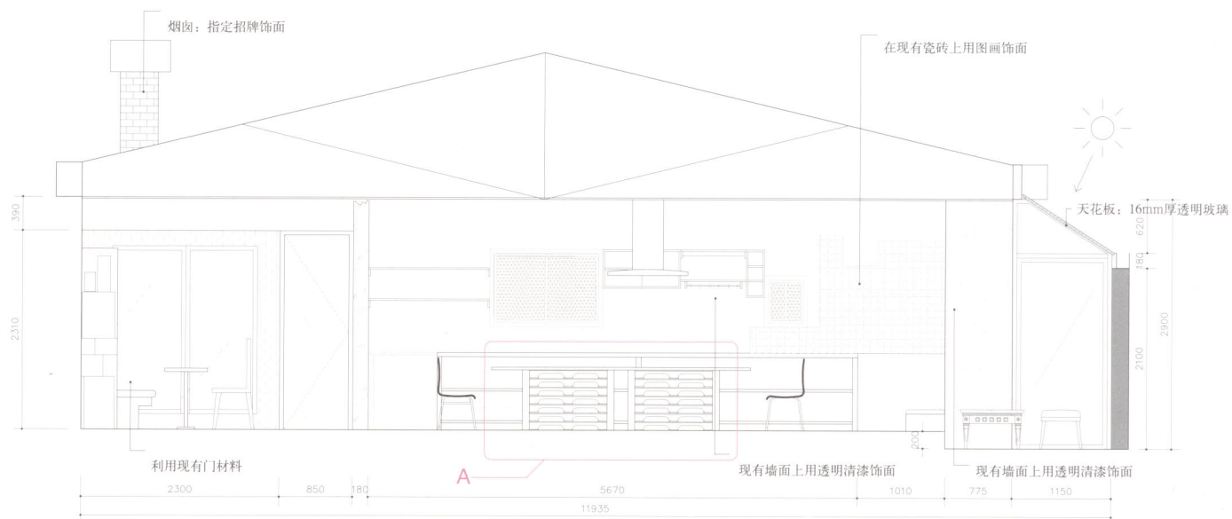
立面图1
