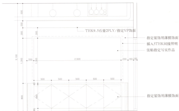
前台细部图
