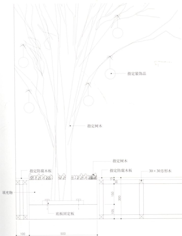
舞台花坛细部图
