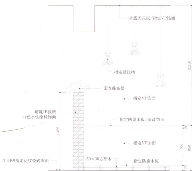
书房细部图
