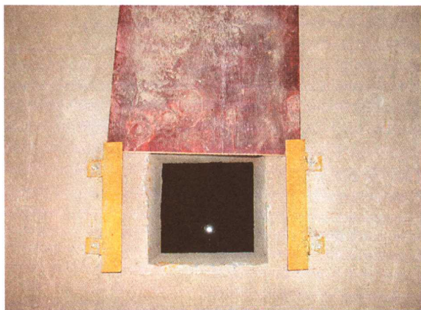
抽拉式施工洞口（上海建工集团）
