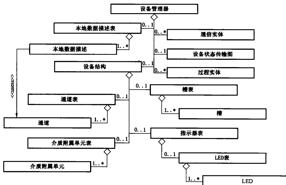
图 6 DeviceManager(设备管理器)分类图
