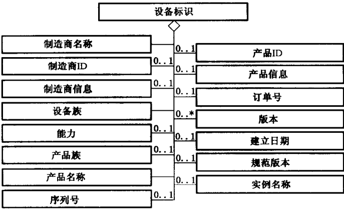
图 5 DeviceIdentity(设备标识)分类图
