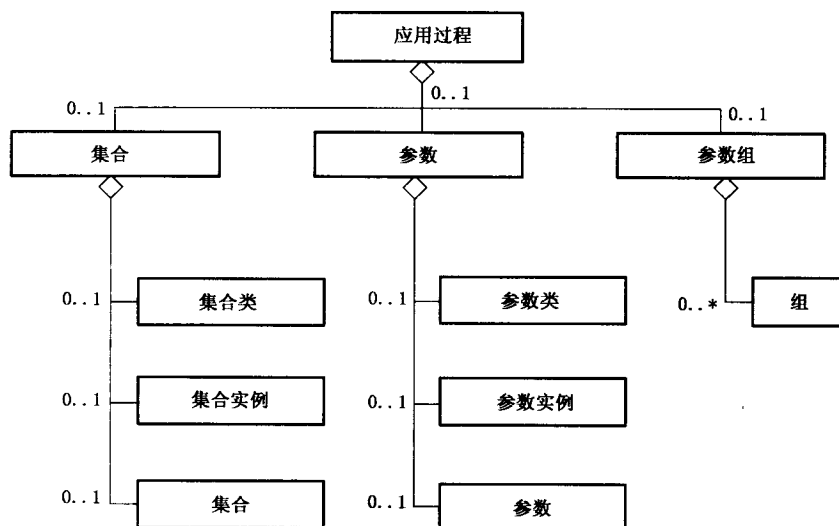
图 2 DeviceNet 应用过程(ApplicationProcess)分类图
