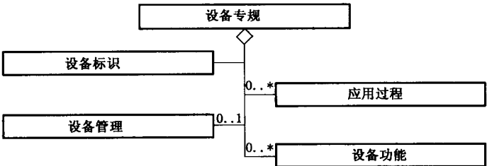
图 4 说明 CANopen 设备专规的分类结构。
