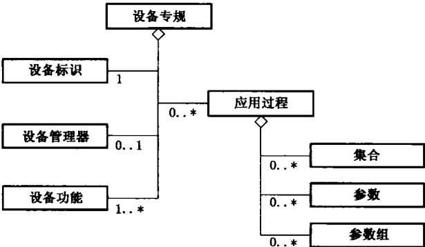
图 1 DeviceNet 设备专规类图
