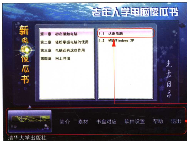
图1 光盘主界面
