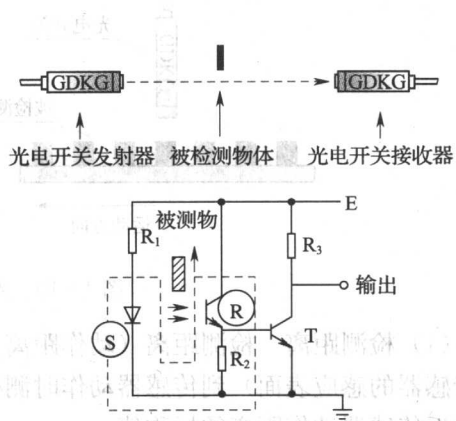
图 1-7 对射式（透射式）光电传感器工作模型示意图
