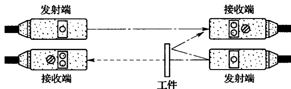
图 1-17 两对透射式传感器并排安装
