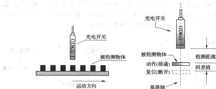
图 1-10 光电传感器术语示意图
