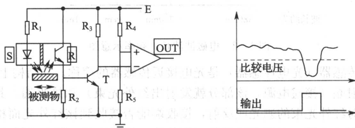
图 1-5 漫反射光电传感器工作模型
