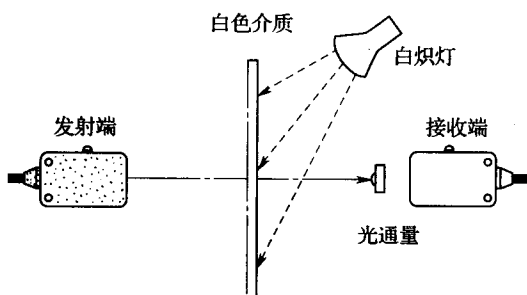
图 1-19 传感器无信号输出或闪烁不定
