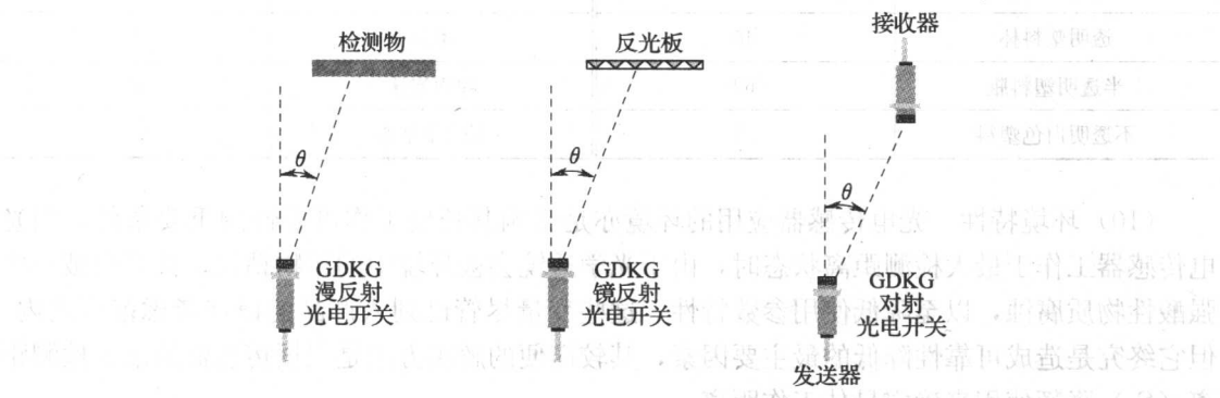
图 1-11 光电传感器的指向角示意图
