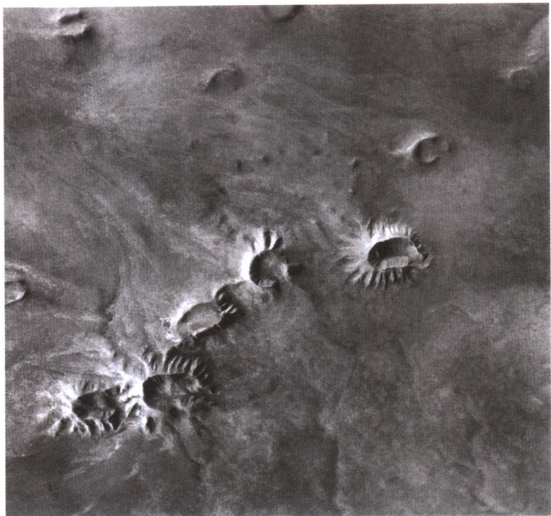
内蒙古锡林郭勒盟灰腾西里熔岩台地上的火山口群（航片）
