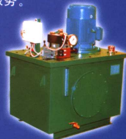
冶金环保设备用液压系统
