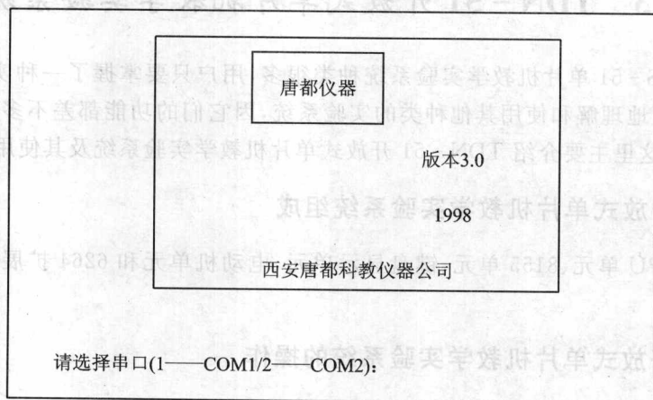
图 1-2 进入系统
