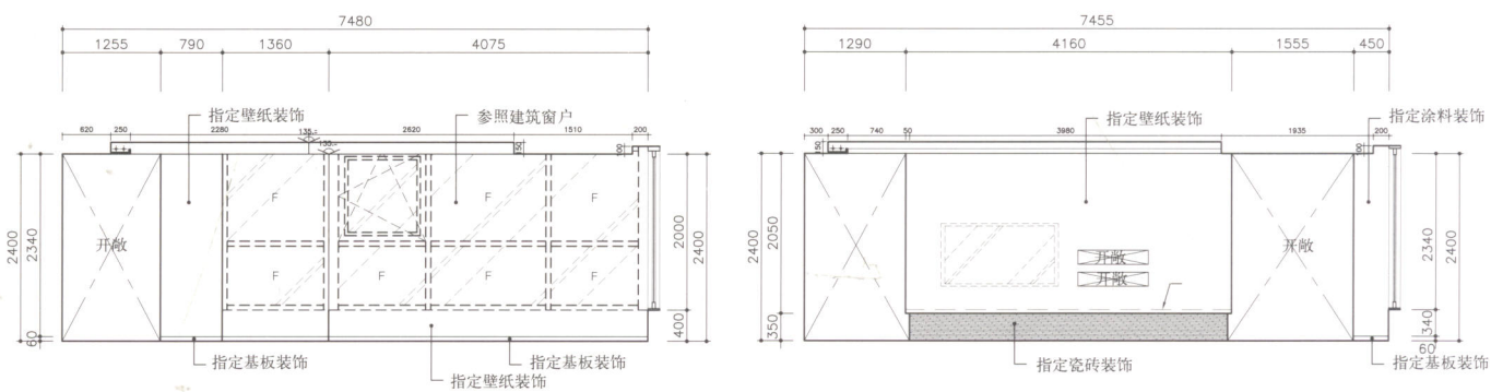
客厅立面图2
