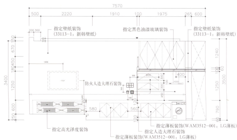
立面图2
