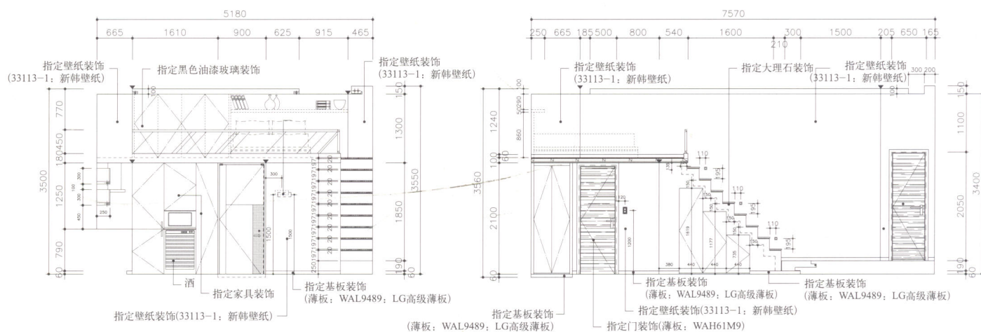
立面图1
