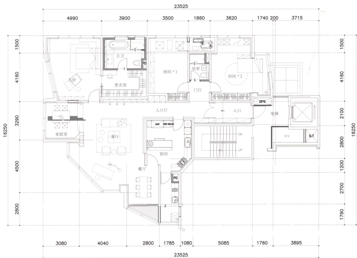
楼层平面图
