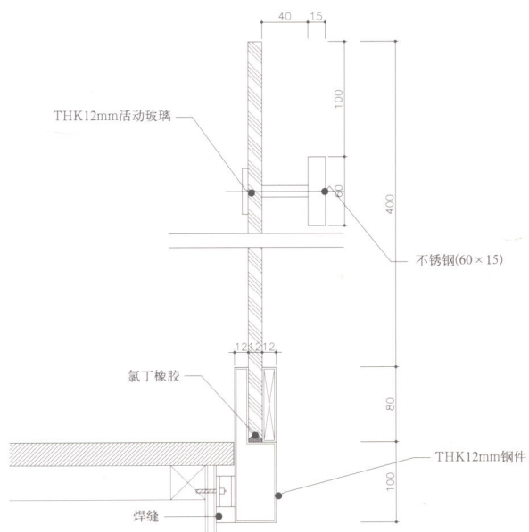
栏杆细部
