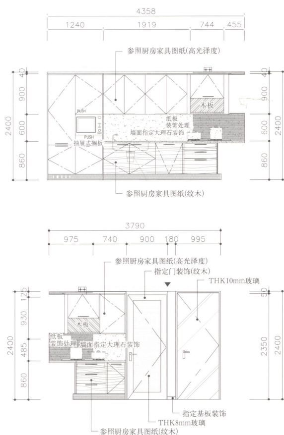
厨房立面图
