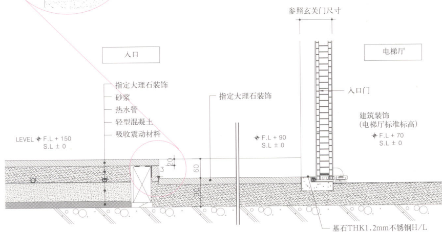
玄关地面截面图
