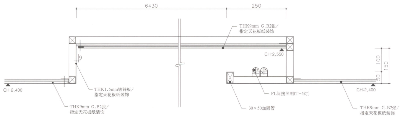
客厅天花板细部
