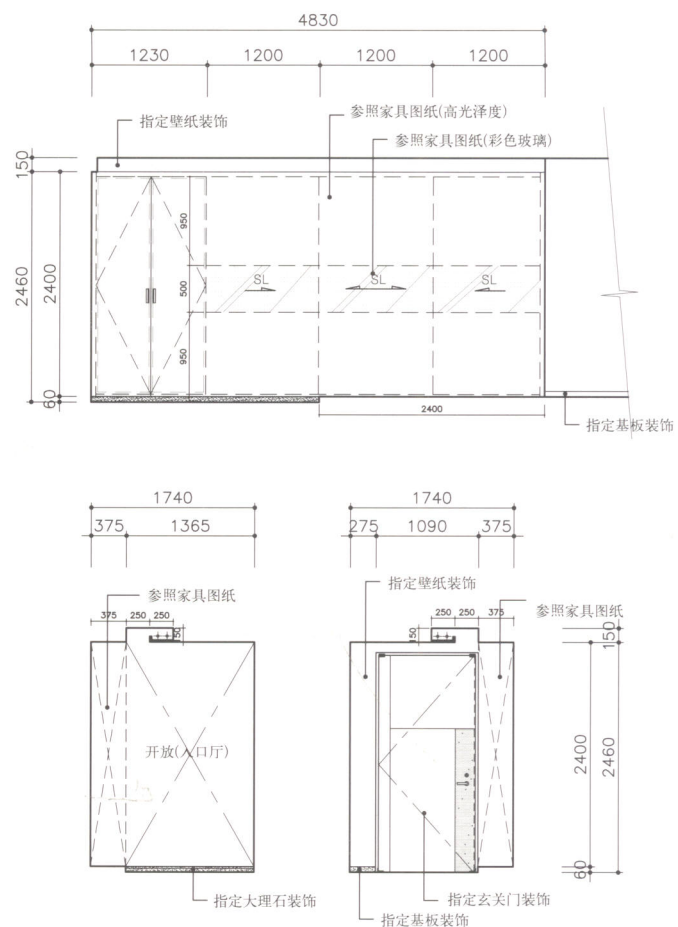
玄关立面图
