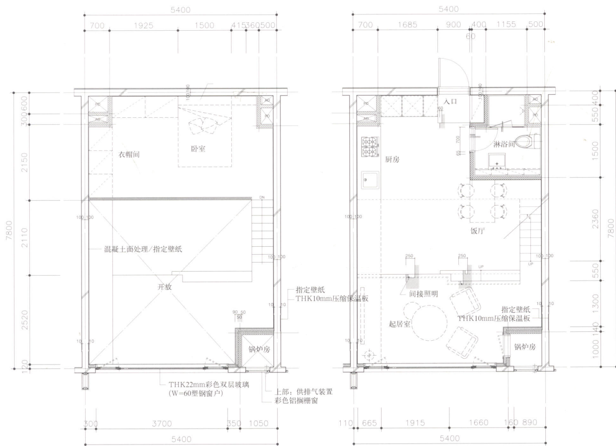
楼层平面图
