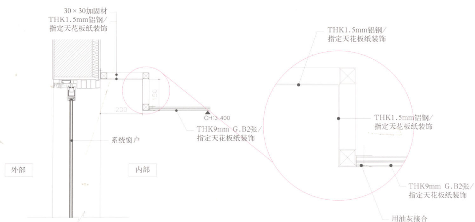
窗帘盒子细部
