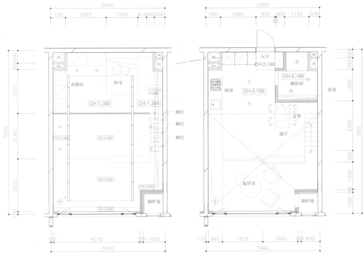
天花板平面图
