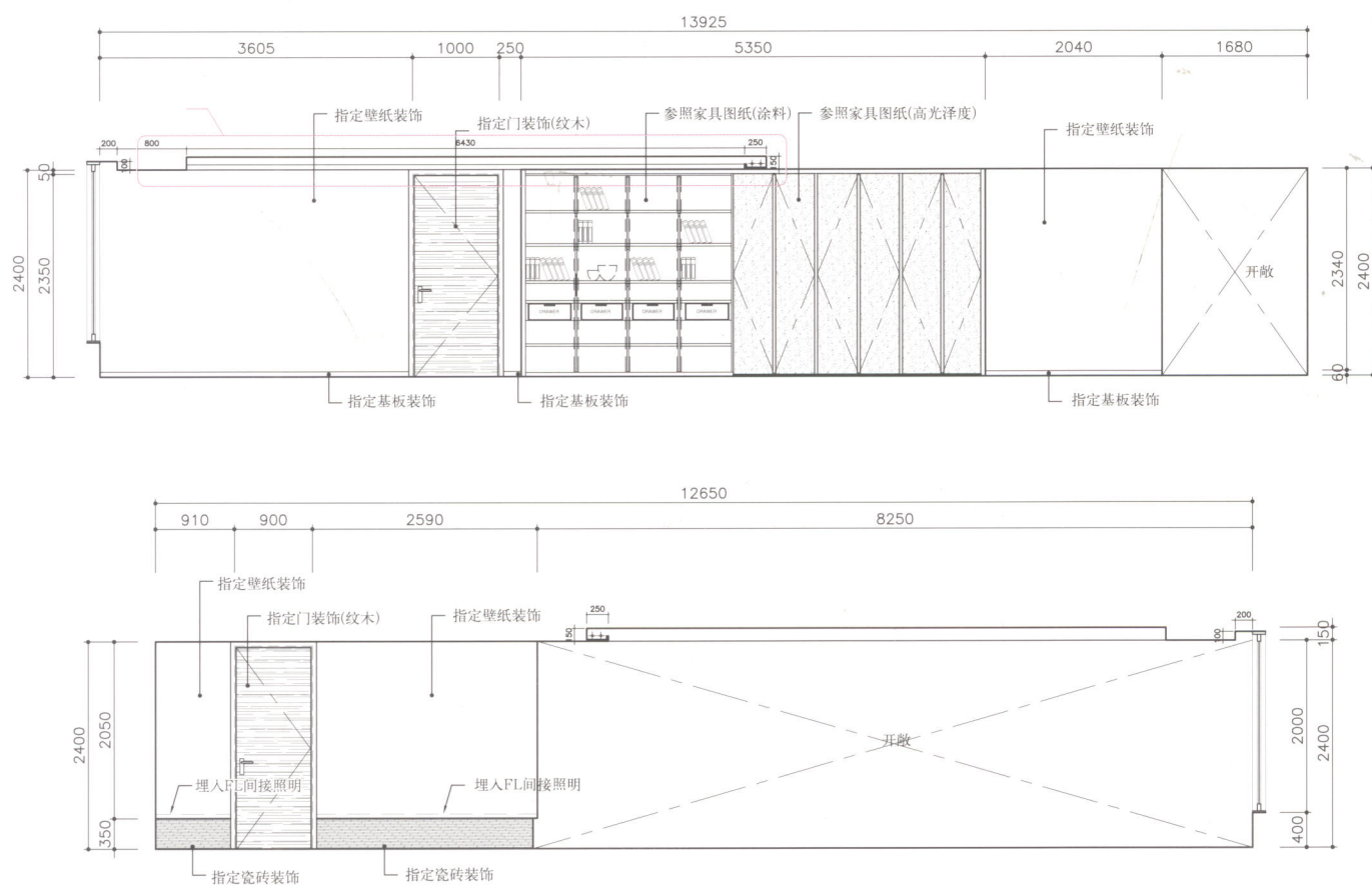
客厅立面图1
