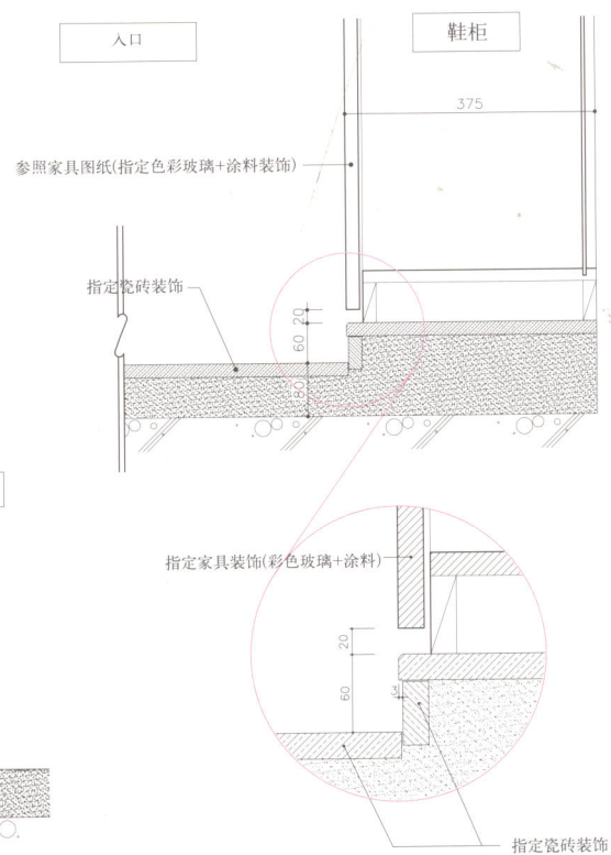
鞋柜地面截面图
