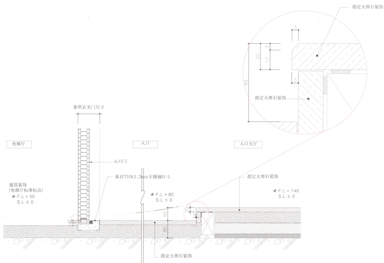
玄关地面细部
