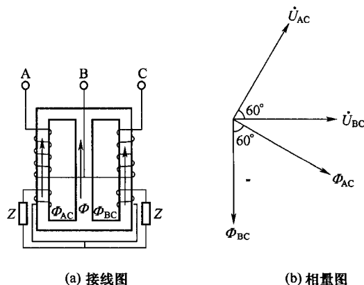
图 2-5 共轭式 V,V 接线原理图
