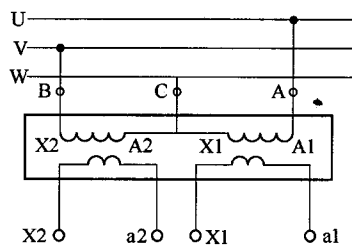
图 2-4 三相 V,V 接线
