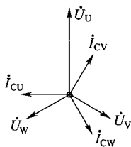
(b) 相量图
