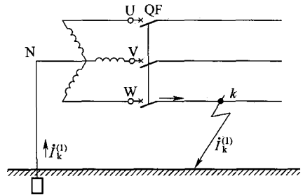
图 1-5 中性点直接接地三相系统
