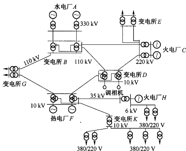
图 1-1 电力系统图
