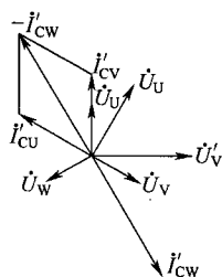
(b) 相量图
