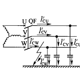
(a) 电路图
