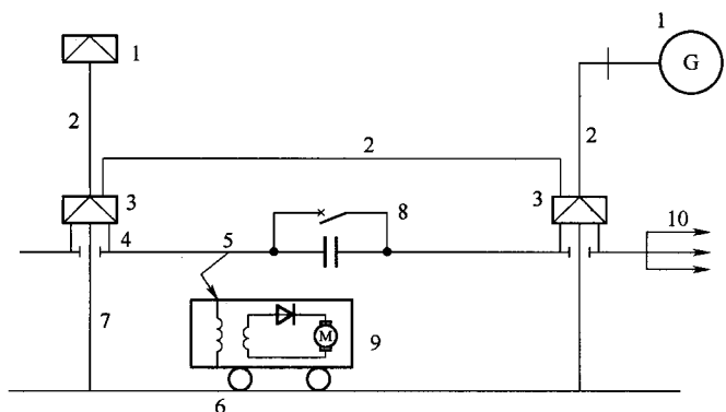
图 2-1 工频单相交流牵引供电系统示意图
