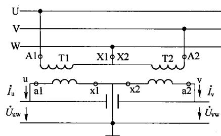
图 2-3 单相 V,V 接线
