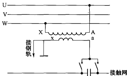
图 2-2 纯单相接线
