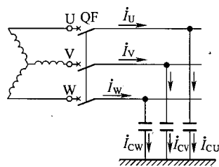
(a) 电路图
