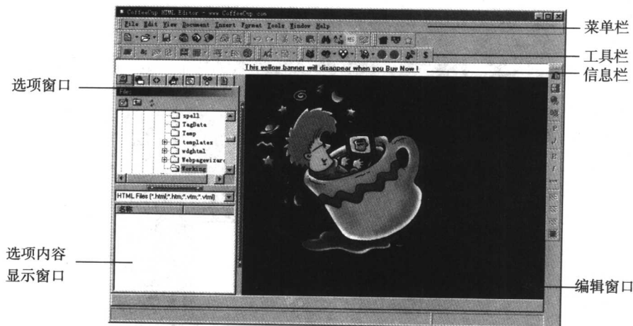
图 1.1 CoffeeCup HTML Editor 的界面
