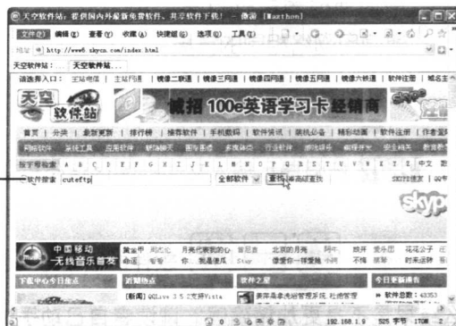
图 1-11 输入关键字
