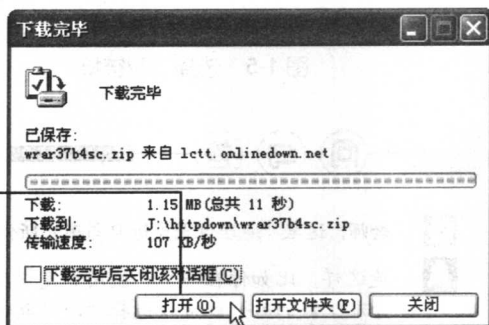
图 1-9 下载完毕
