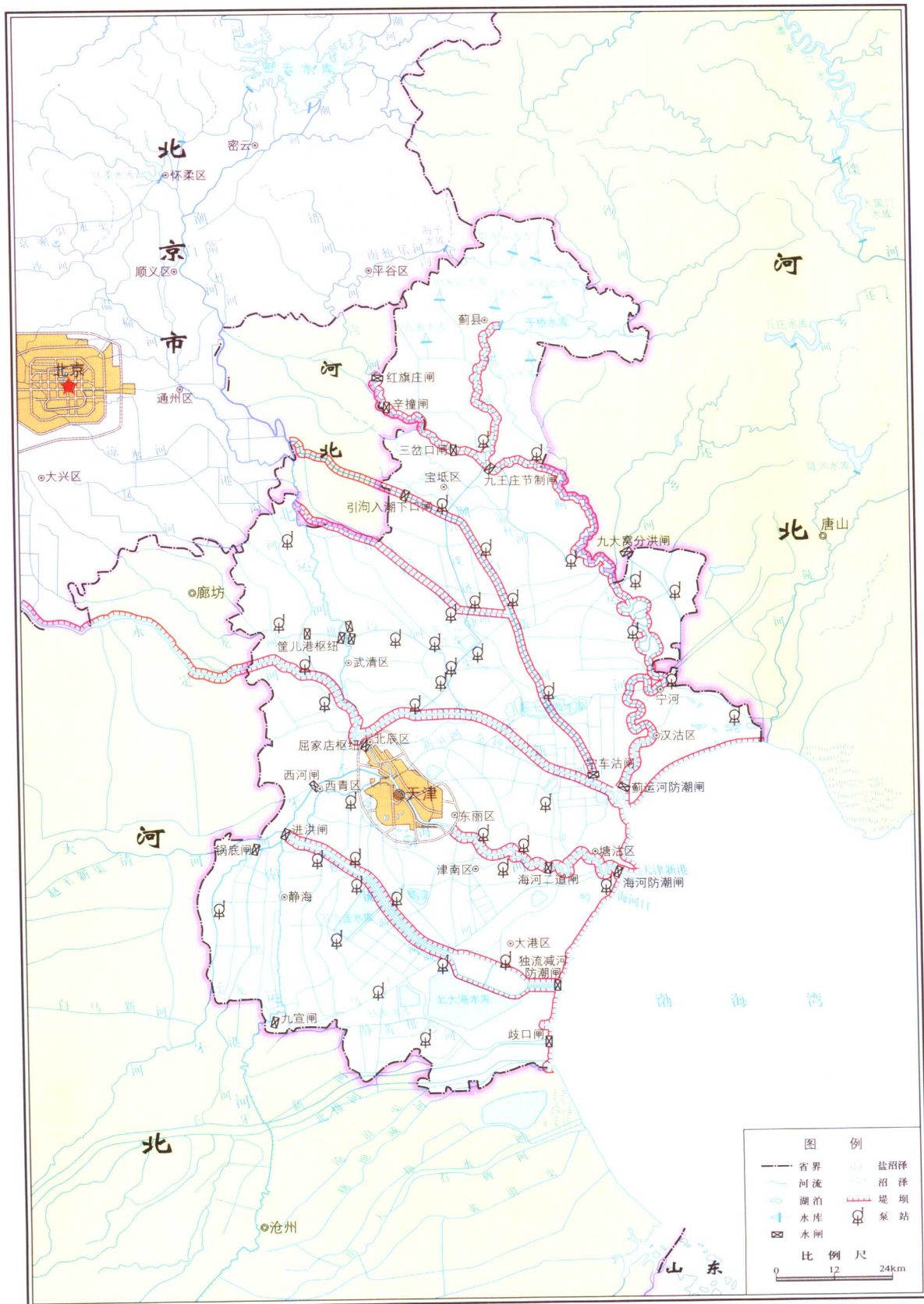
2. 天津市水系及工程分布示意图
