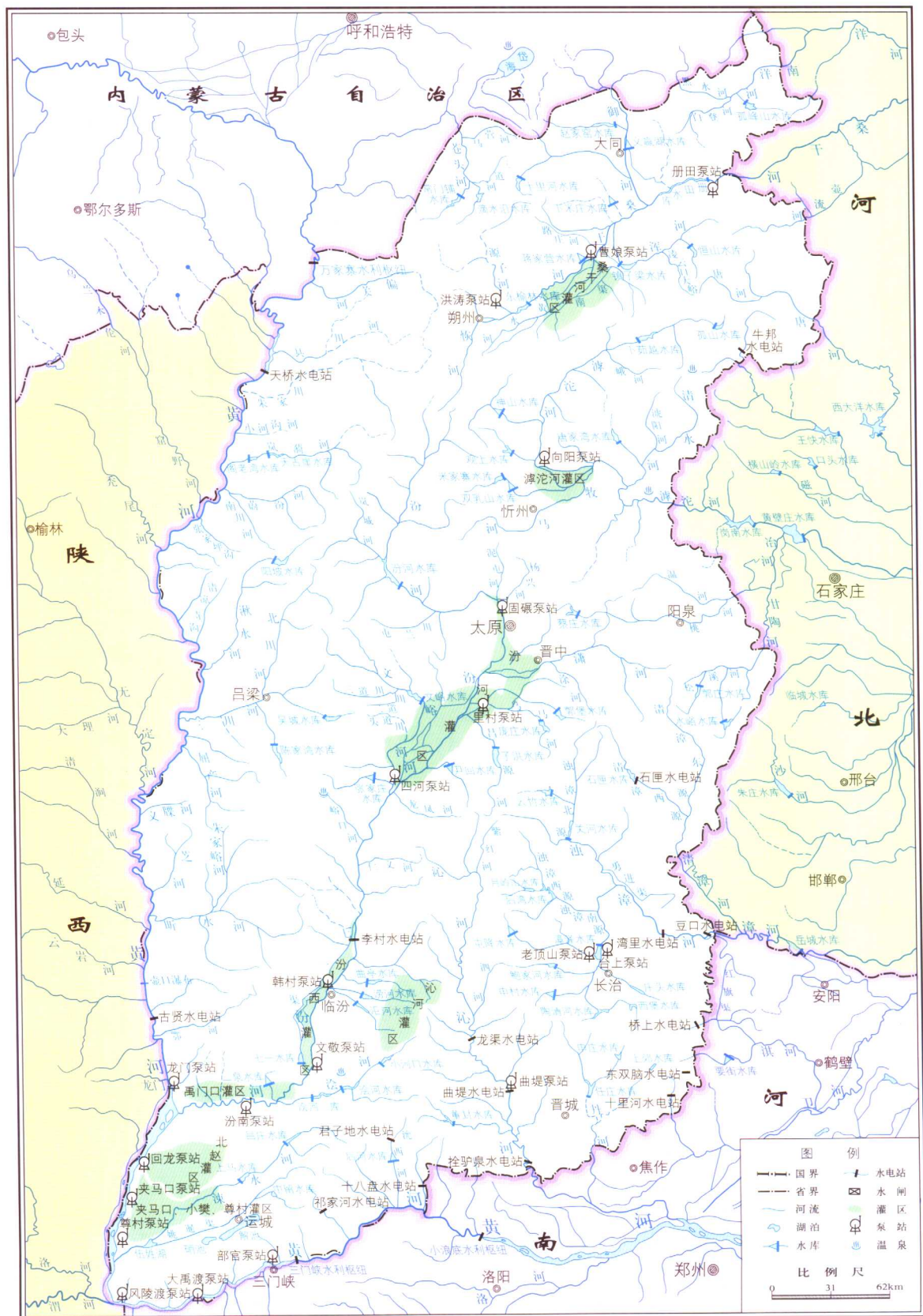
4. 山西省水系及工程分布示意图
