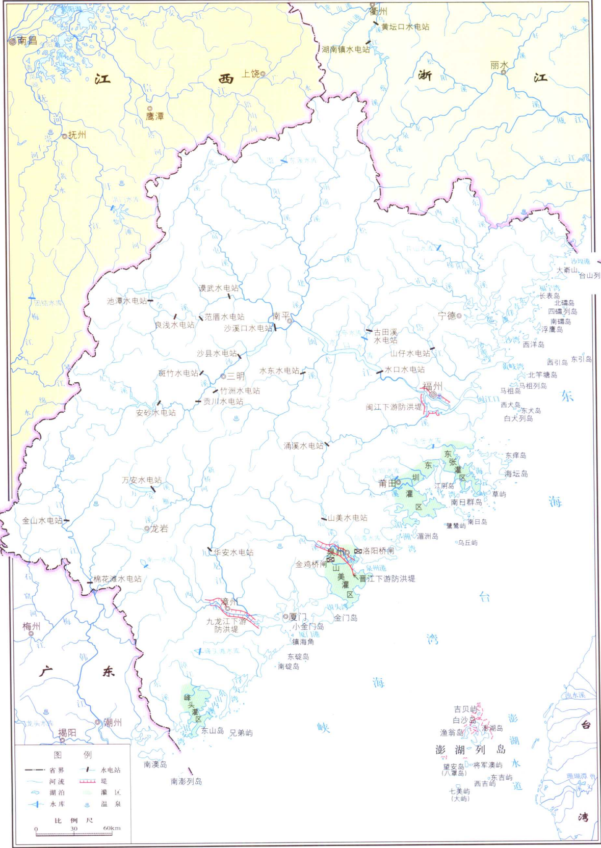
13. 福建省水系及工程分布示意图
