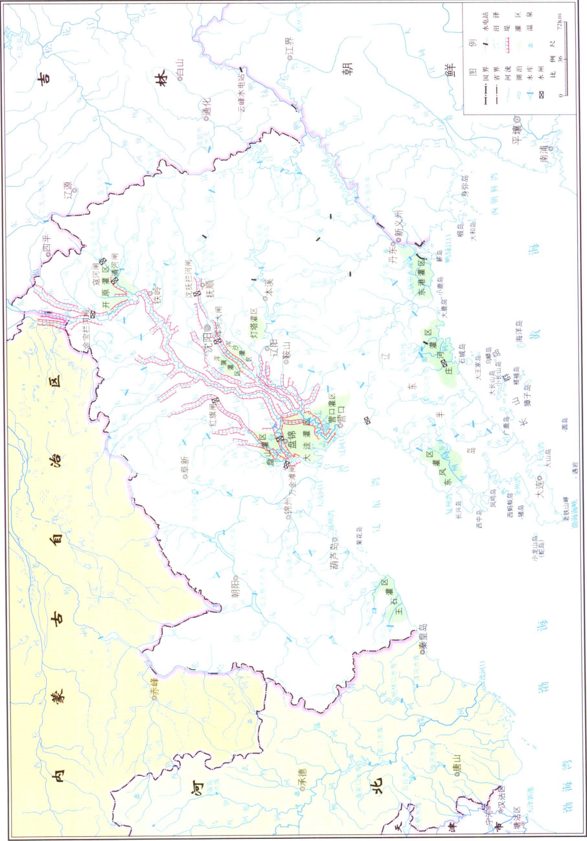
6. 辽宁省水系及工程分布示意图
