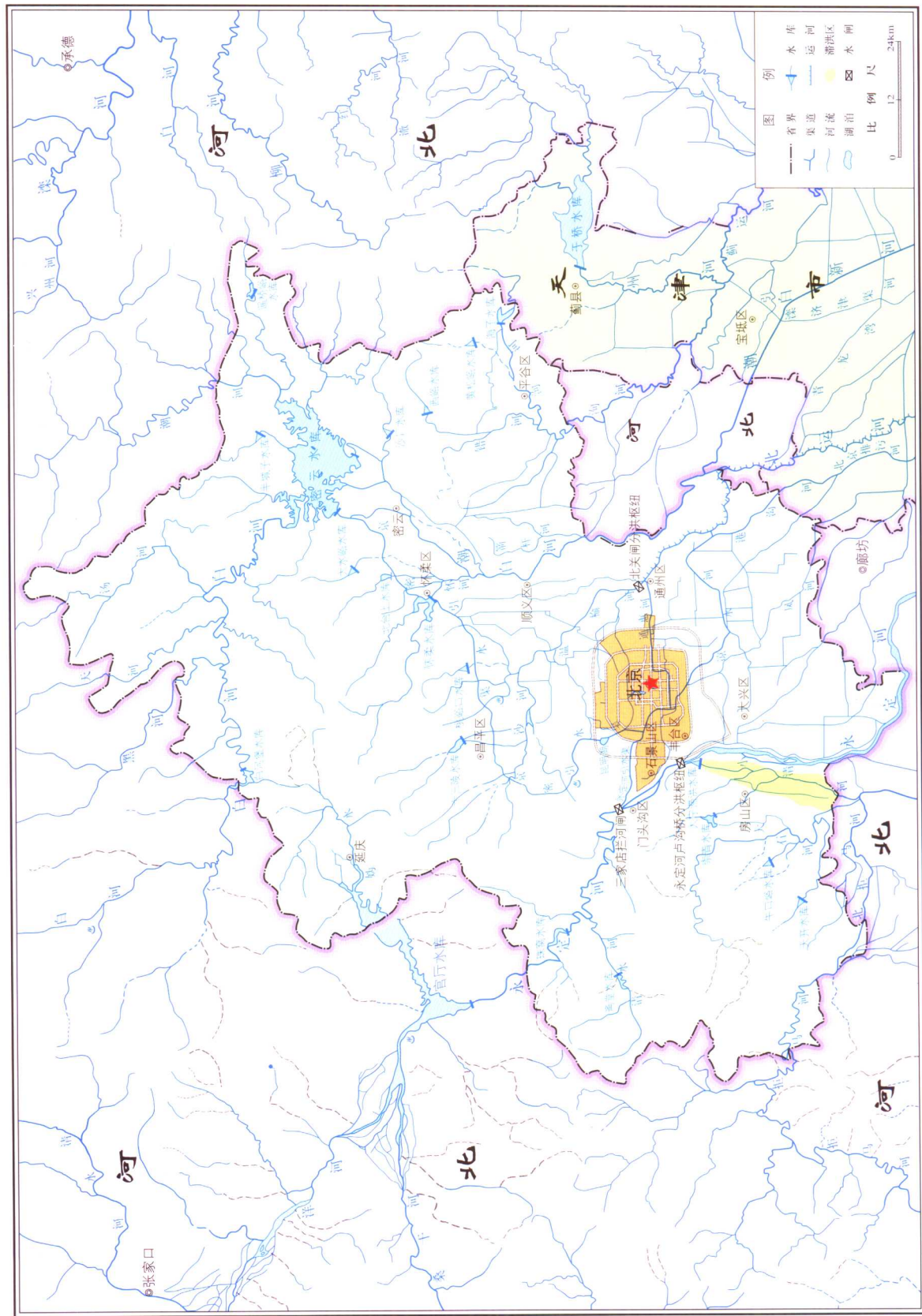
1. 北京市水系及工程分布示意图
