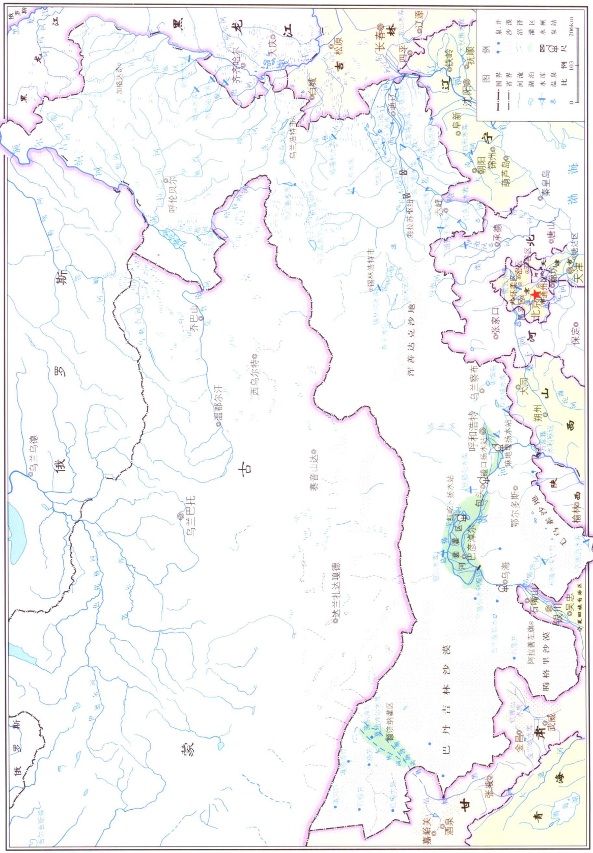
5. 内蒙古自治区水系及工程分布示意图
