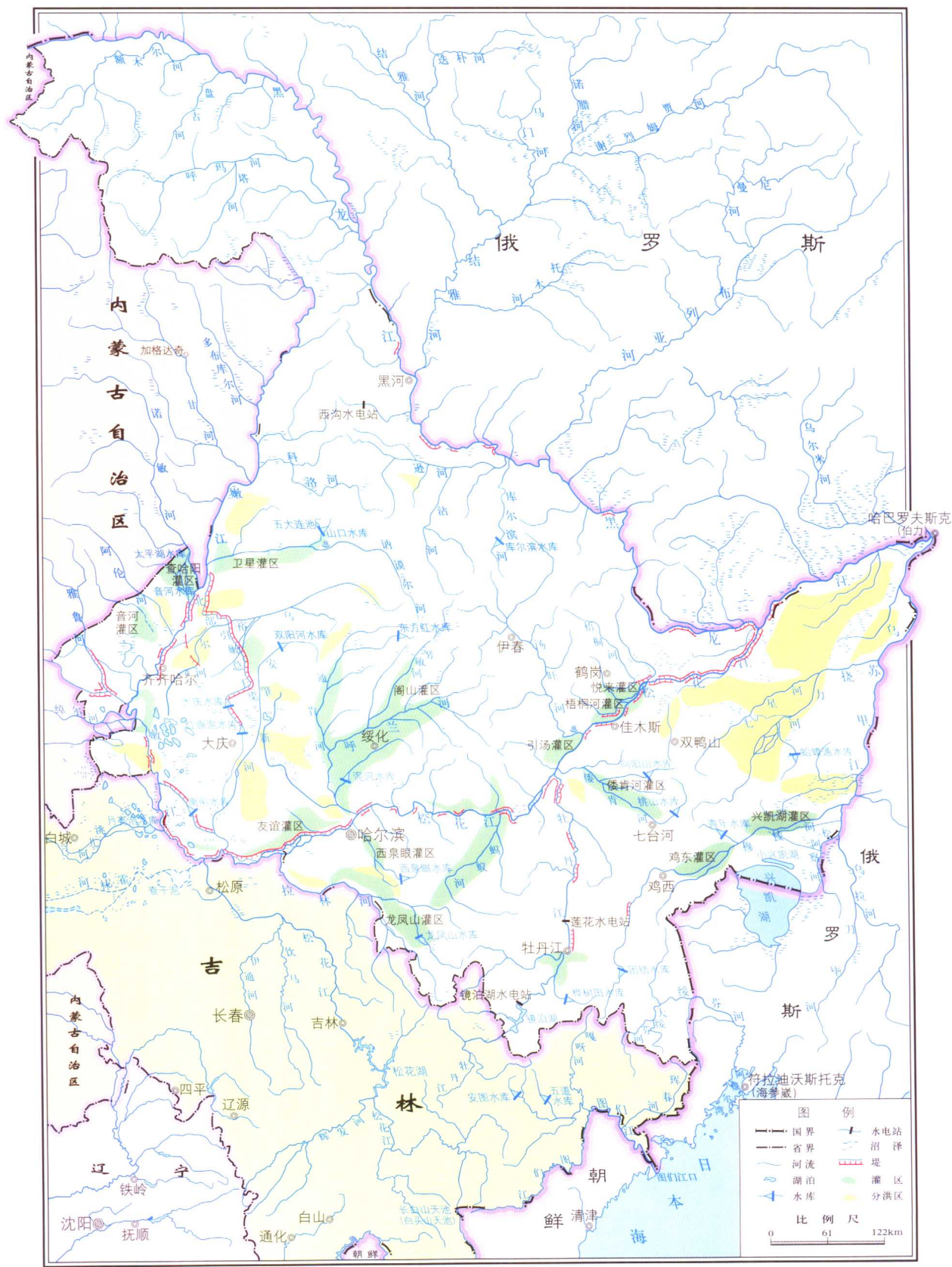
8. 黑龙江省水系及工程分布示意图
