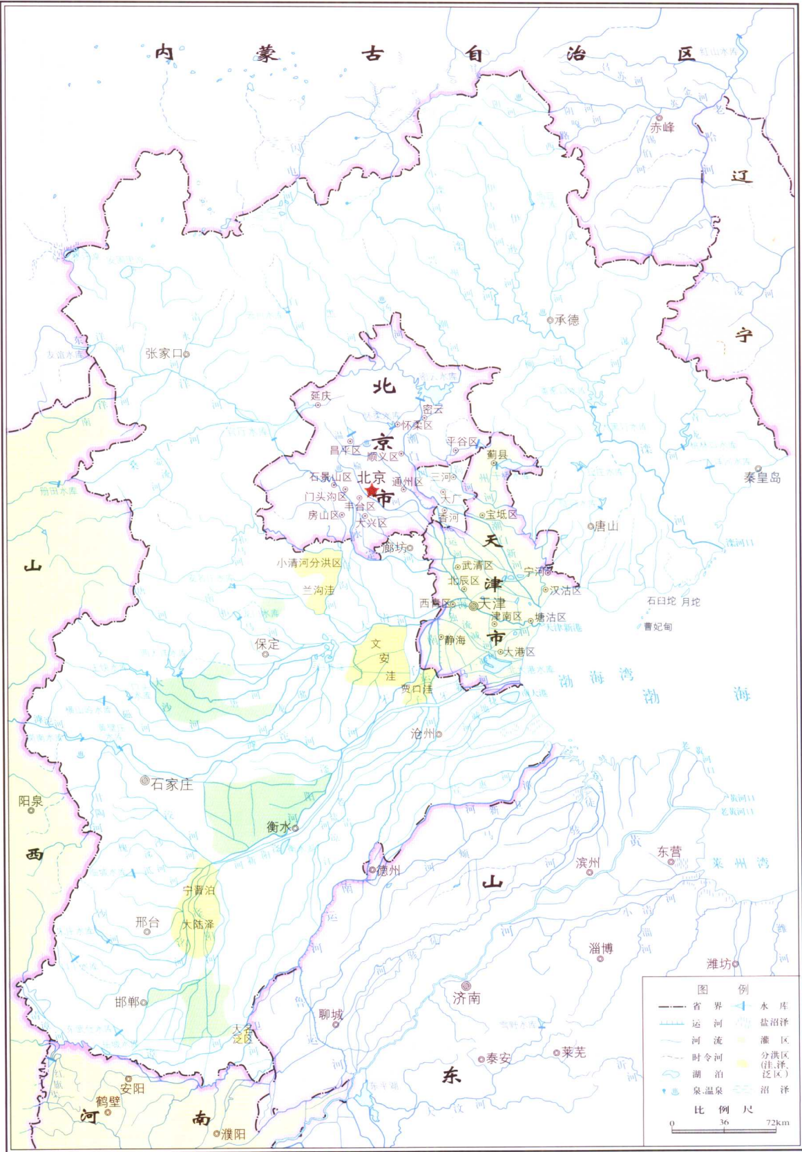
3. 河北省水系及工程分布示意图
