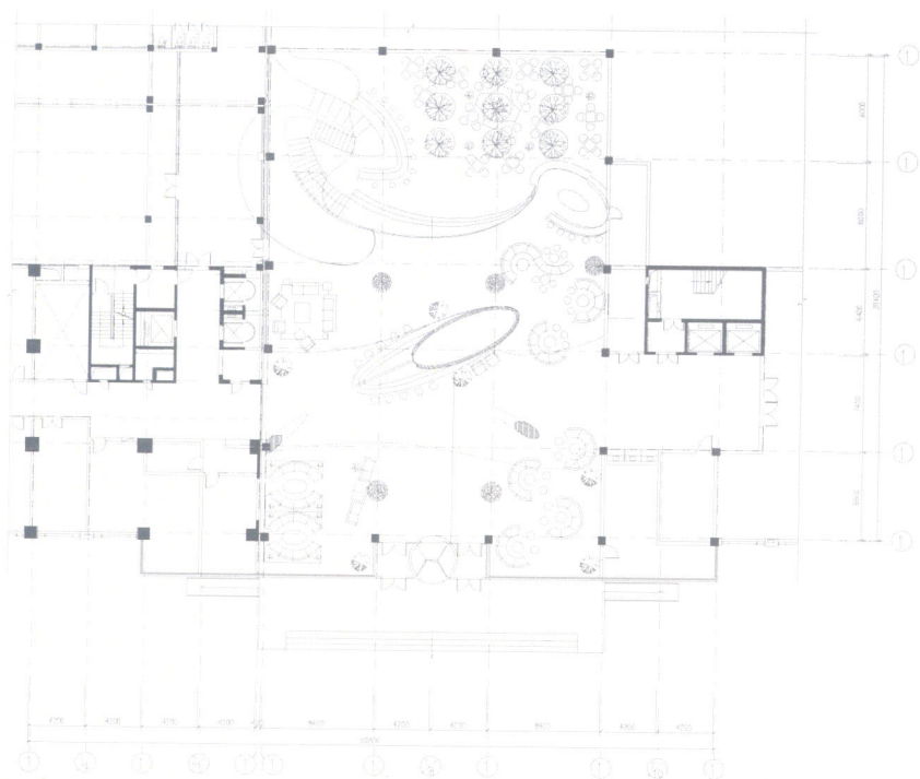
一层平面图
