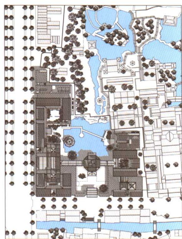
庭院平面图
