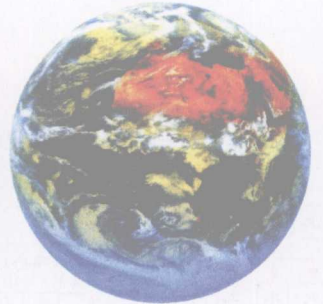
从人造地球卫星上拍摄的地球照片
