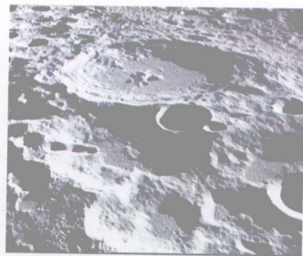
月球环形山
