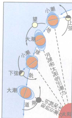
潮汐的形成
