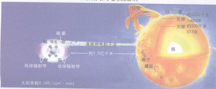
太阳活动对地球的影响
