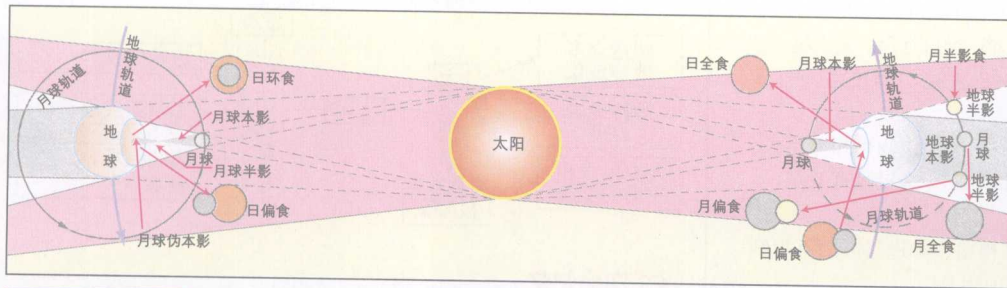
日食和月食的成因
