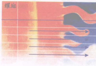
太阳活动对地球的影响
