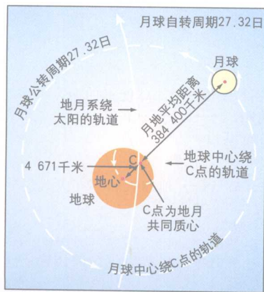
地月系运动
