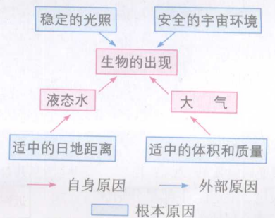
地球适于生物生存的条件
