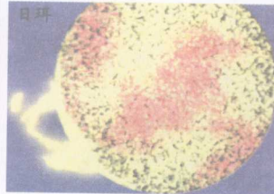
主要太阳活动
