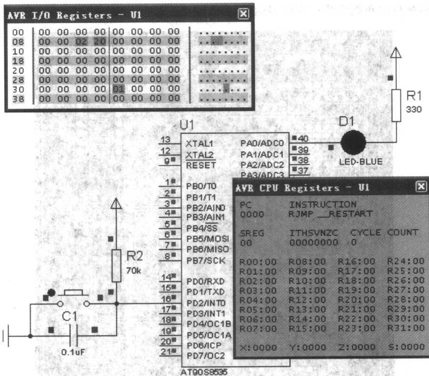
图 1-7 微处理器电路仿真
