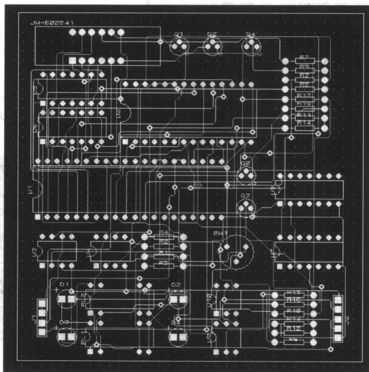
图 1-9 PROTEUS PCB 布线
