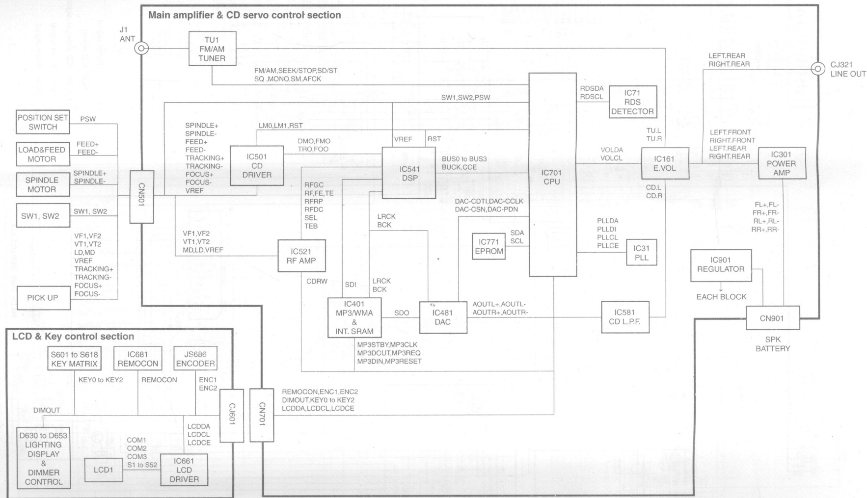
框图
