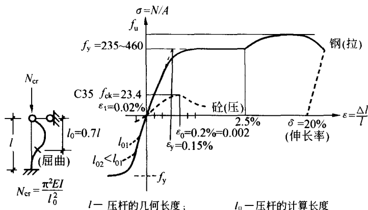
图 1-1 钢和砼 \sigma-\epsilon 曲线的比较
