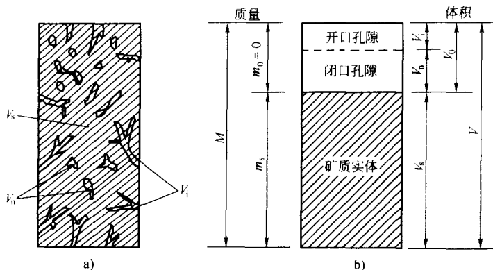
图 1-1 岩石组成结构示意图
