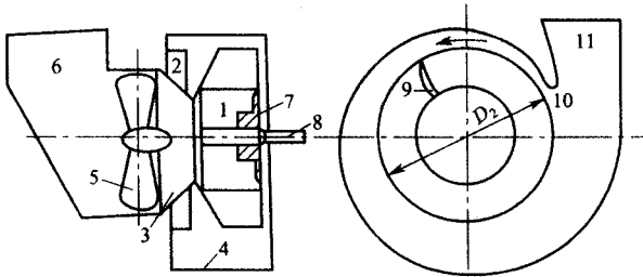
图 2-2 离心通风机结构示意图
