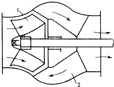
图 2-4 混流式泵简图
