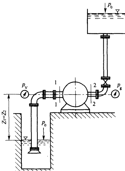
图 2-6 扬程的确定
