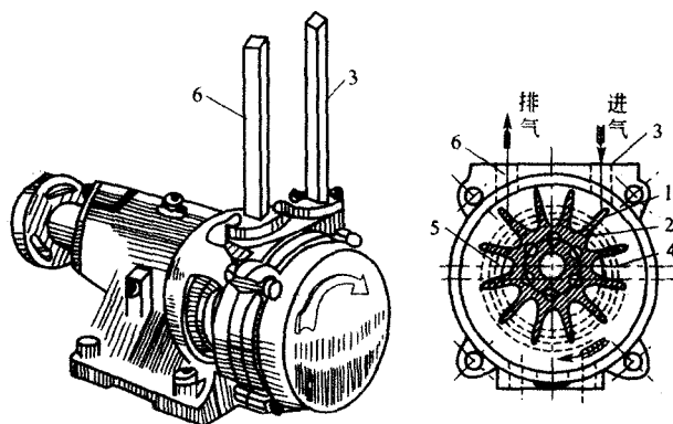
图 2-5 水环式真空泵结构示意图
