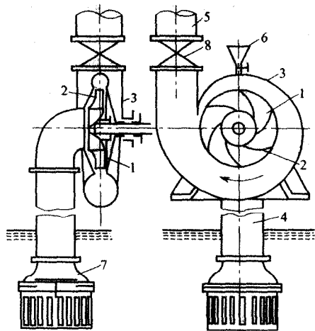
图 2-1 离心泵工作简图
