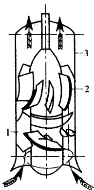
图 2-3 轴流泵简图
