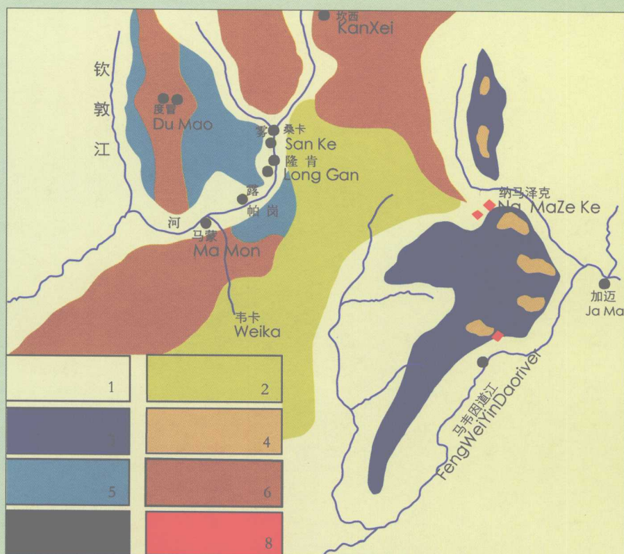
缅甸北部含翡翠的地质构造示意图
