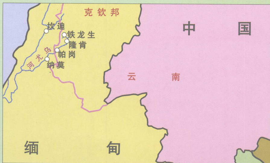
缅甸翡翠主要产地雾露河（乌尤河）流域示意图
