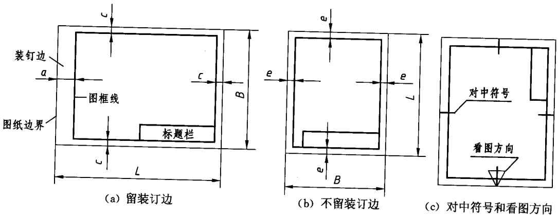
图 1-2 图框格式和看图方向
