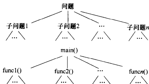
图 1-1 自顶向下的功能分解与程序结构
