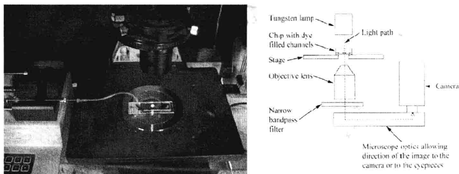
Fig. 5. Apparatus
