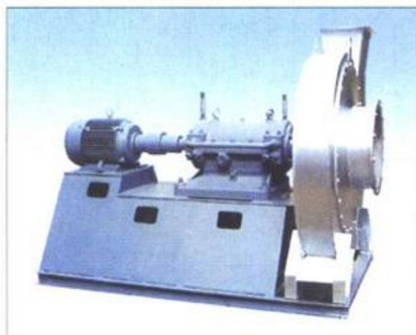
FW9-26 系列高温防腐离心通风机
