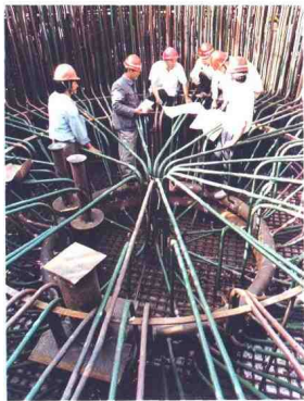
建设中的国家“863”高技术项目——高温气冷堆
