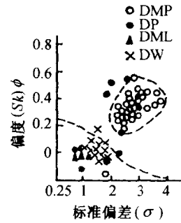
图 2 偏度与标准偏差散点
