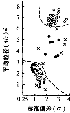
图 1 平均粒径与标准偏差散点
