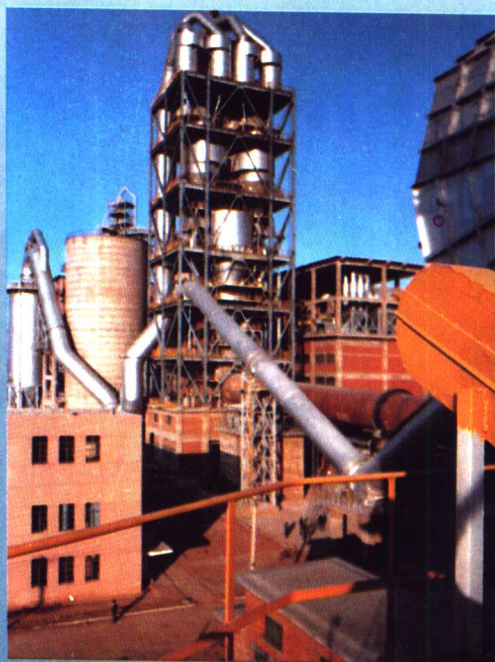
窑尾予热器
