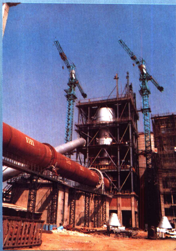
200 T M自升塔式起重机
