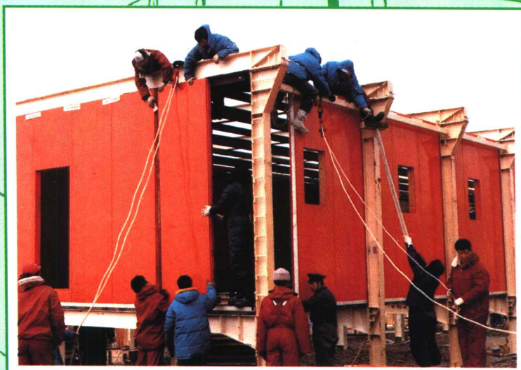
安装外墙板
