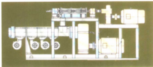
MD50、75、100 连续密炼机
