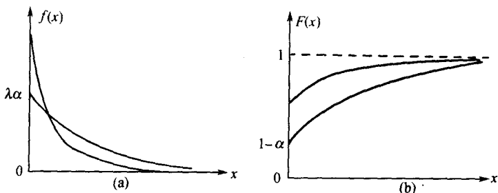
图 1.1 指数分布族的密度函数与分布函数
