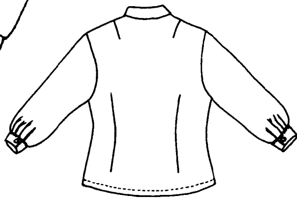
图 1-4 女衬衫基本款式后视图
