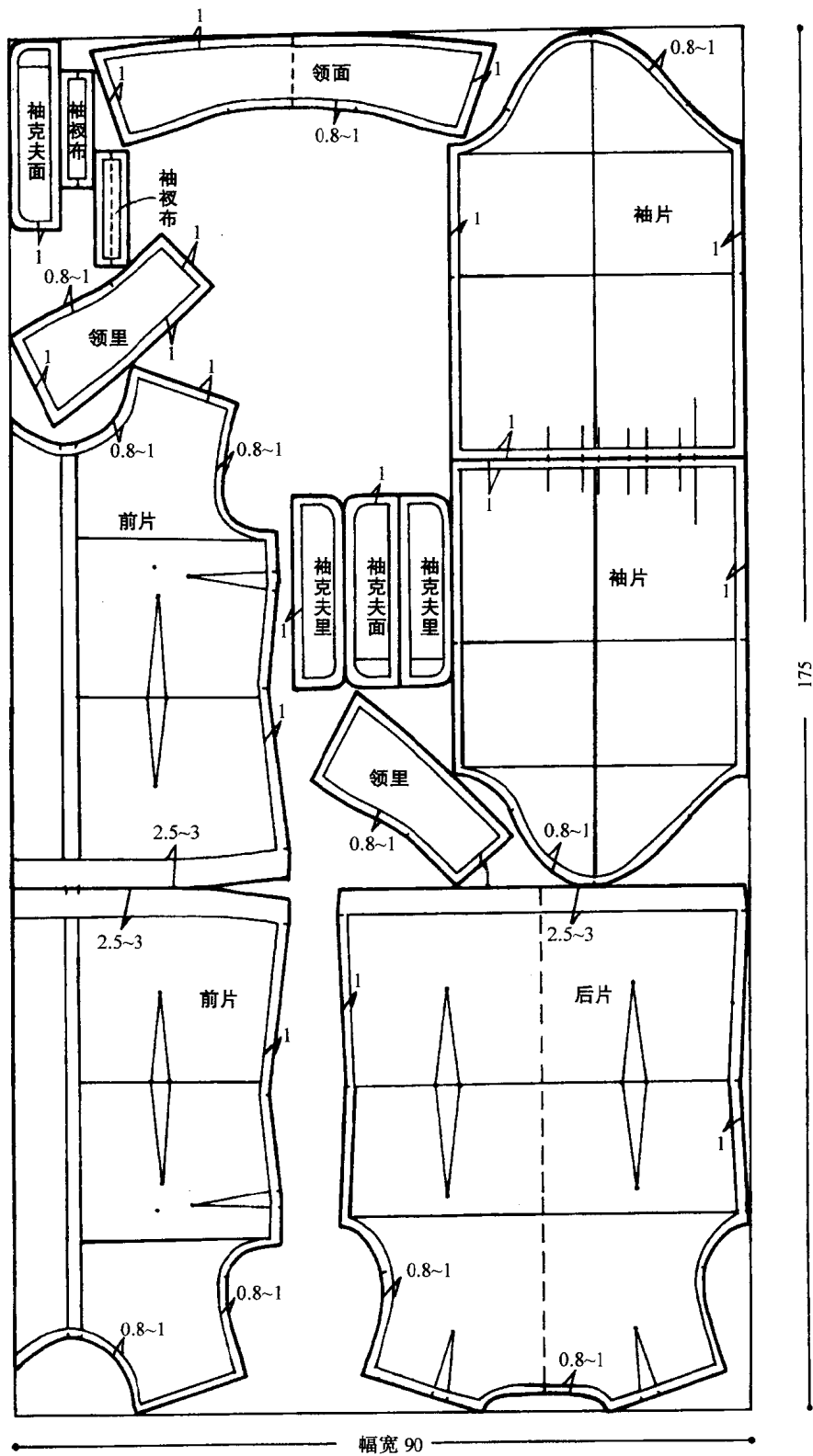
图 1-6 女衬衫基本款式排料方法一
