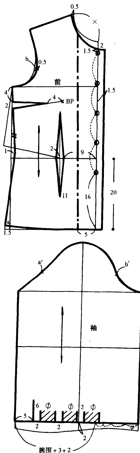
图 1-5 女衬衫基本款式的裁剪图
