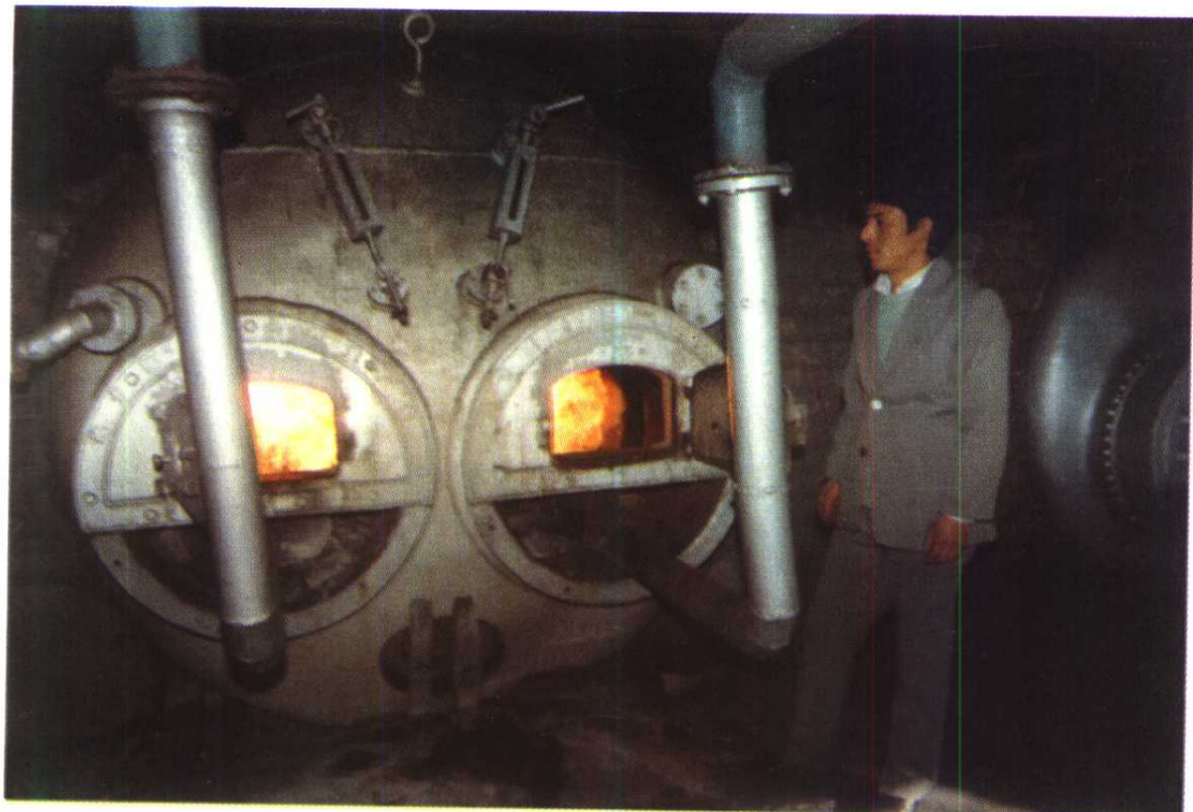
包头矿务局河滩沟矿利用抽放的瓦斯烧锅炉
