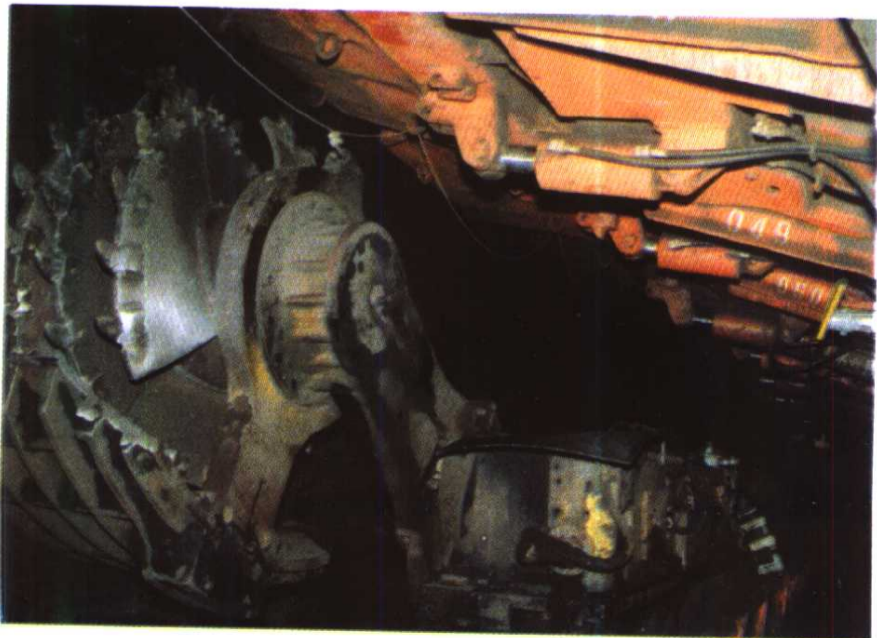
大雁矿务局综采工作面
