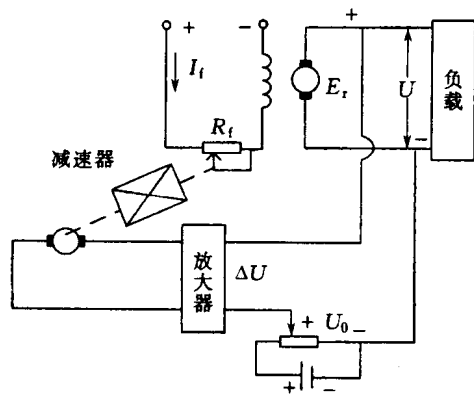
图 1.5 闭环控制
