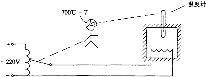
图 1.1 手动控制电加热炉
