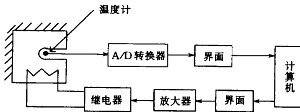
图 1.7 炉温的计算机控制系统
