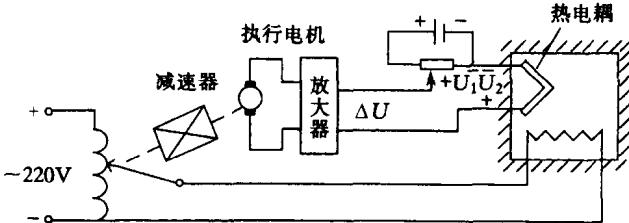
图 1.2 自动控制电加热炉
