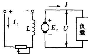
图 1.4 供电系统
