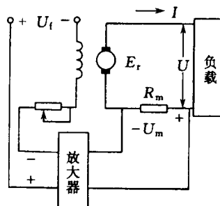
图 1.6 前馈控制系统
