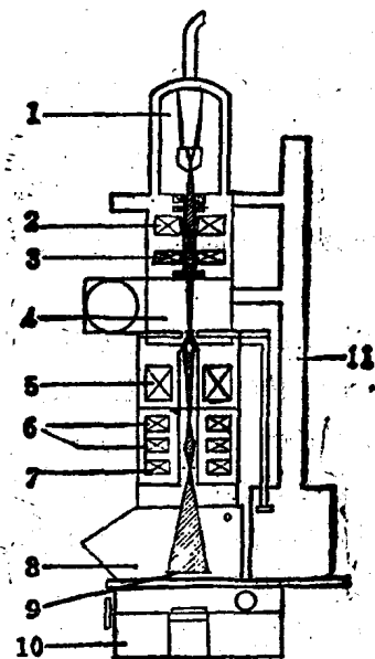
图 2 电子显微镜原理示意图
