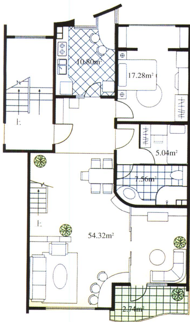
底层平面
