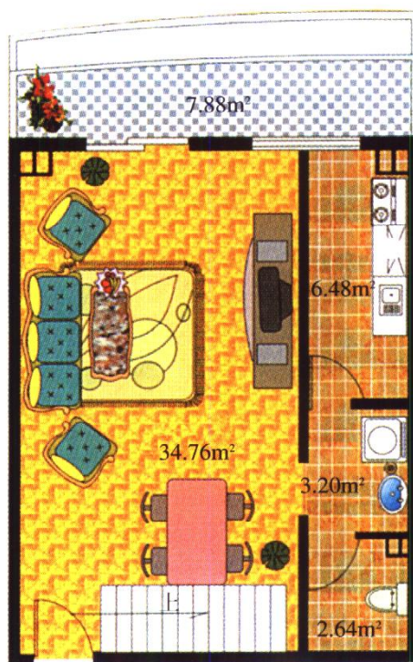
一层平面
