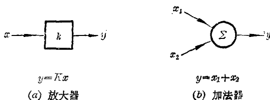
图 0-3 理想运算器
