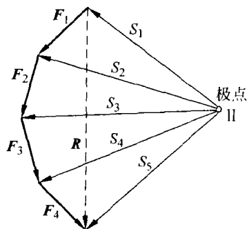
力多边形
