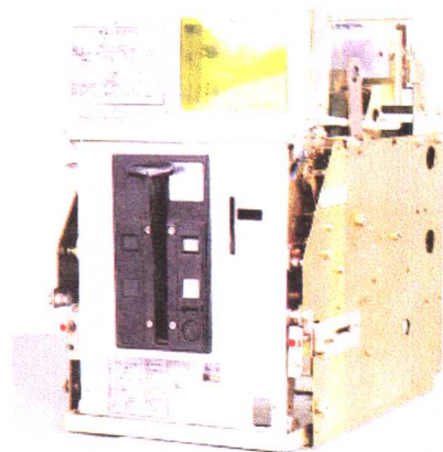
DW914 (AH) 船陆两用低压空气断路器
