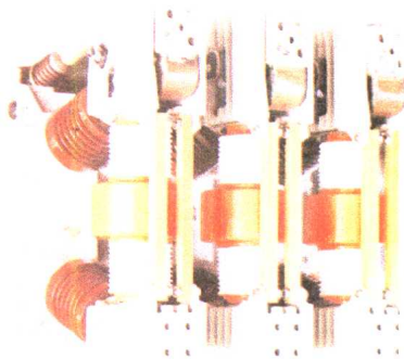
ZN12-10 型系列户内 高压真空断路器
