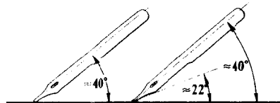
笔尖头整形后与纸面的倾斜角
