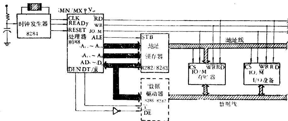
图1.5 最小方式系统的结构
