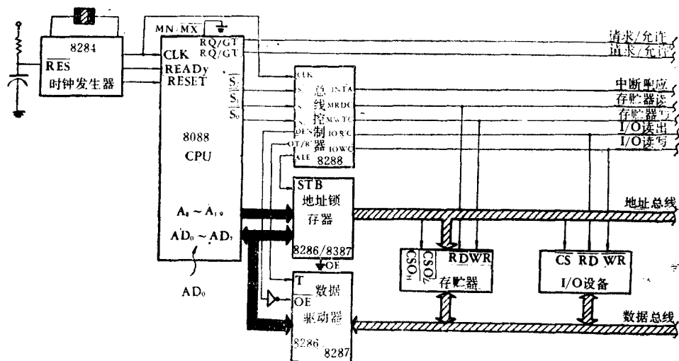
图1.6 IBMPC最大方式系统的组成
